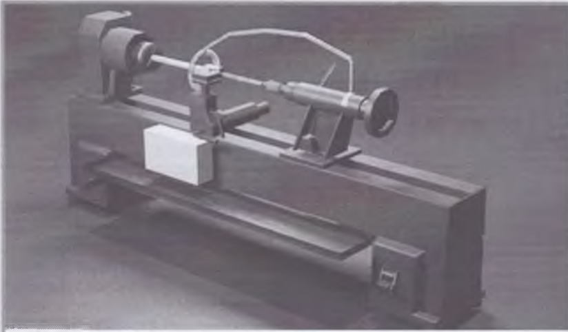
Рис. 2. Расположение электромагнитной катушки при обработке детали на токарном станке
