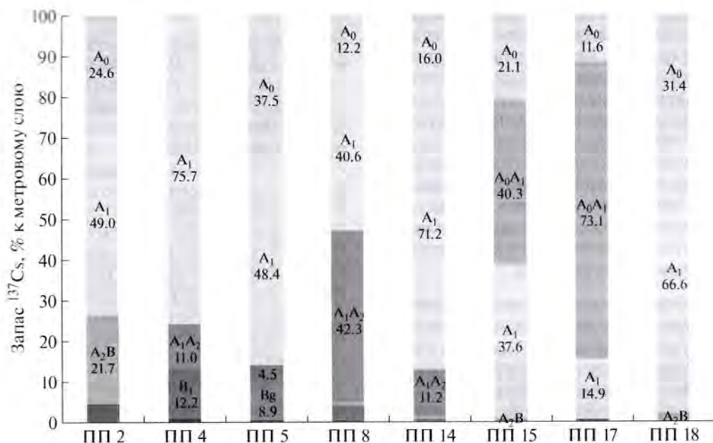
Рис. 3. Распределение ^{137}\text{Cs} в профиле почв сосново-березовых фитоценозов. ПП 2 – среднередкая слабоподзолистая легкосуглинистая почва на моренных отложениях, перекрытых покровным суглинком; ПП 4 – слабоподзолистая легкосуглинистая почва на моренных отложениях, перекрытых покровным суглинком; ПП 5 – среднередкая слабоподзолистая легкосуглинистая глееватая почва на моренных отложениях, перекрытых покровным суглинком; ПП 8 – слабодерновая слабоподзолистая со следами оглеения легкосуглинистая почва на покровном суглинке; ПП 14 – среднередкая слабоподзолистая легкосуглинистая почва на флювиогляциальных песках с прослойками морены; ПП 15 – среднередкая слабоподзолистая песчаная почва на флювиогляциальных песках с прослойками морены; ПП 17 – среднередкая среднеподзолистая супесчаная почва на морене; ПП 18 – среднередкая среднеподзолистая супесчаная почва на морене.
